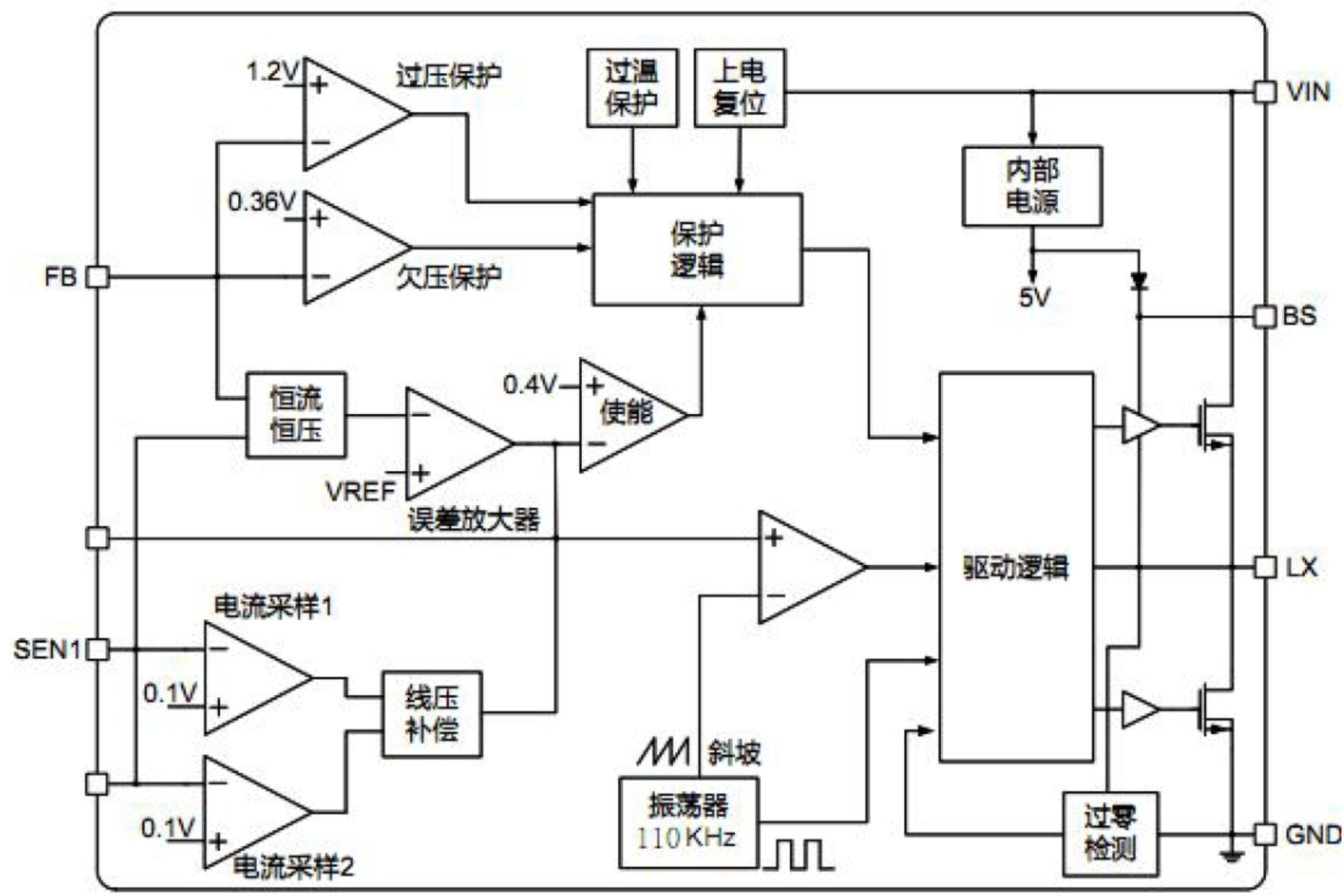
GC1850 内部功能框图
