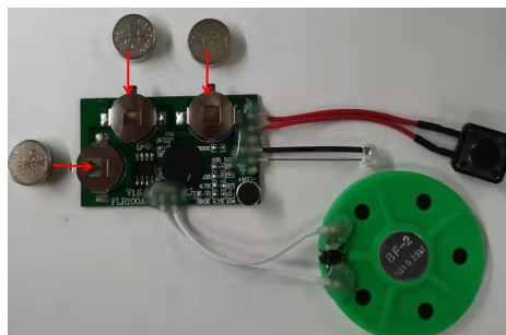
AG13 电池安装，将 3 个分别插入对应电池座
